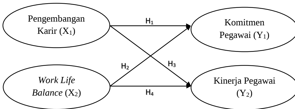
Gambar 1 Kerangka Pikir
